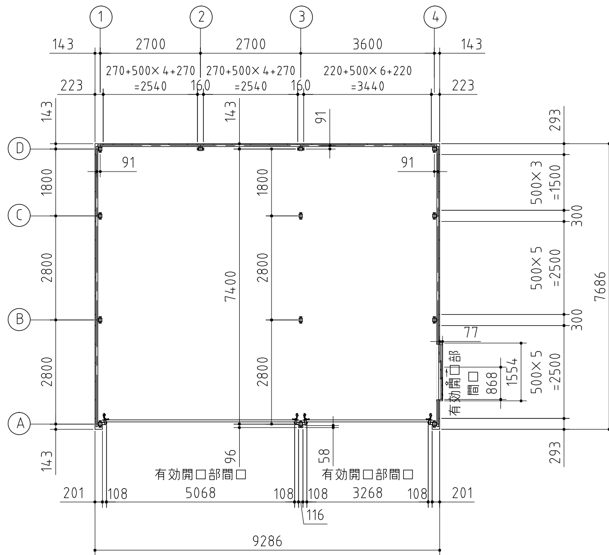
平面図
